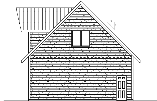
RIGHT ELEVATION SCALE: 1/4" = 1'-0"
